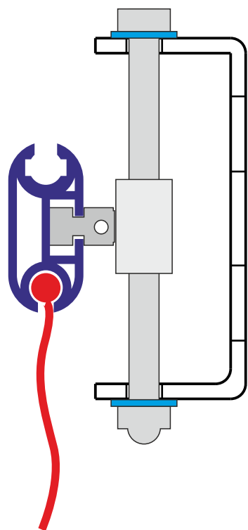
Profil 45/20 Alu - 600cm
